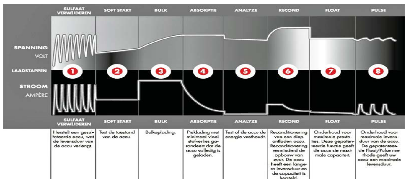
Het laadverloop in 8 stappen van de Ctek druppellader XS 800
